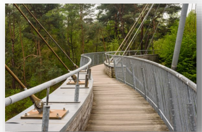
S-vormige voetgangersbrug
